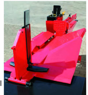
Fließende Übergänge vom Spaltkanal zum Spalttisch
